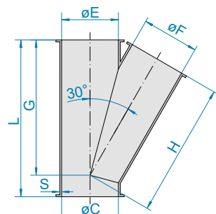
■ Lateral 30°
