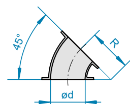
Cast-iron segment 45°
